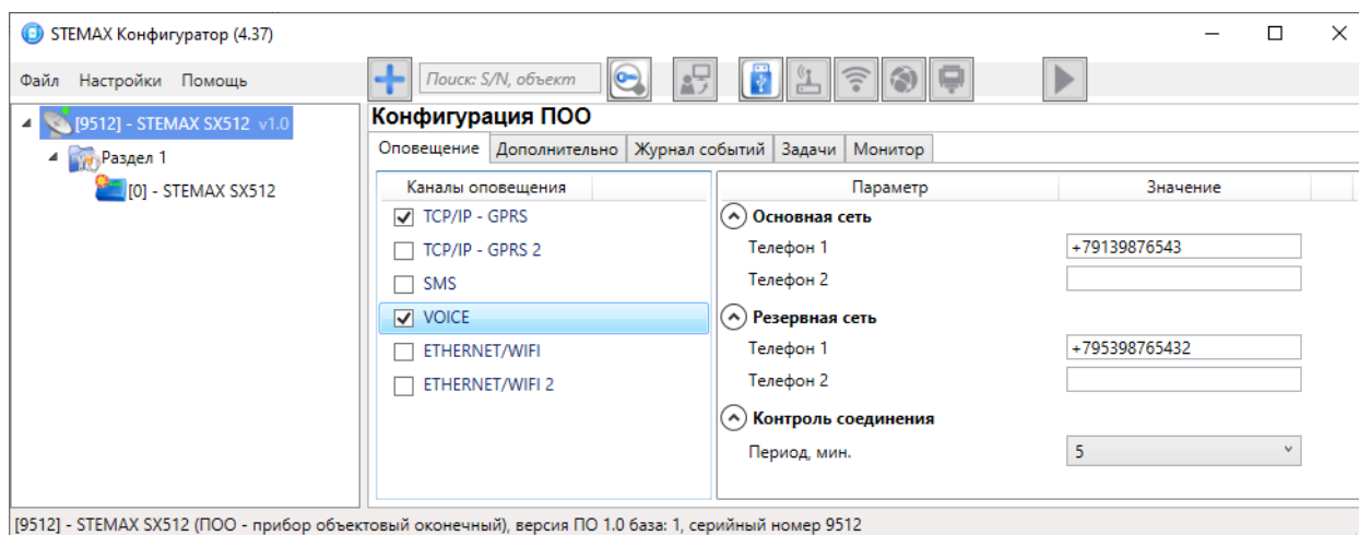
Рисунок 4.20 — Параметры канала Voice
