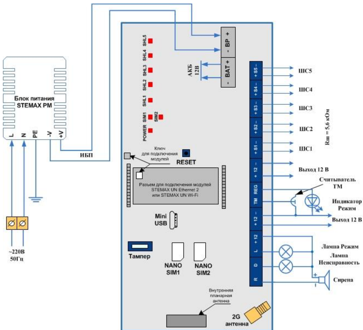
Рисунок А.1 — Схема внешних подключений контроллера
