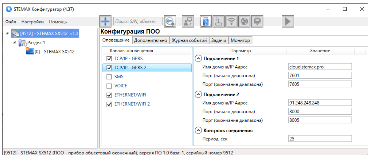
Рисунок 4.18 — Параметры канала TCP/IP GPRS 2
