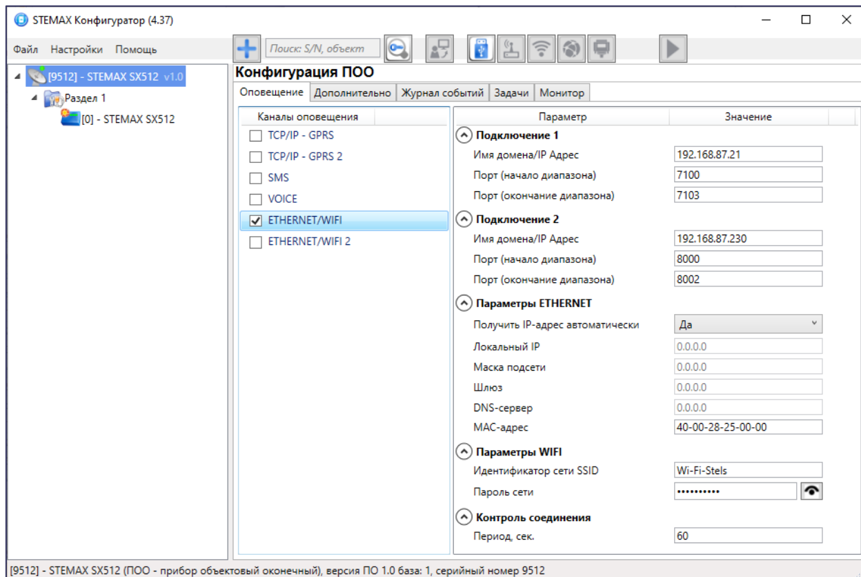
Рисунок 4.21 — Параметры канала ETHERNET/WIFI
