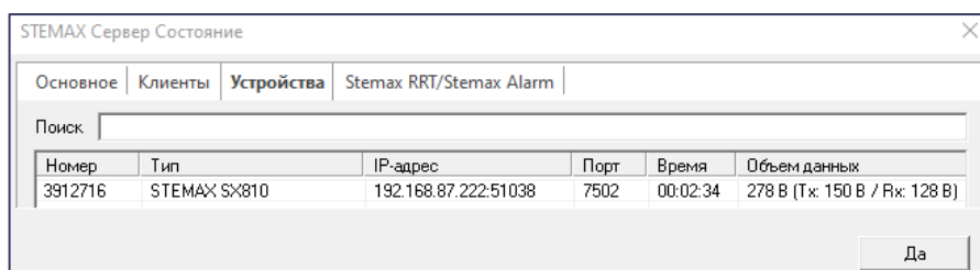
Рисунок 4.13 — Состояние сервера STEMAX
