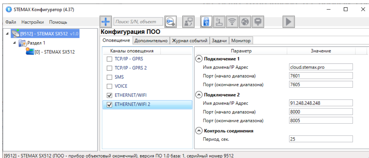
Рисунок 4.22 — Параметры канала TCP/IP GPRS 2
