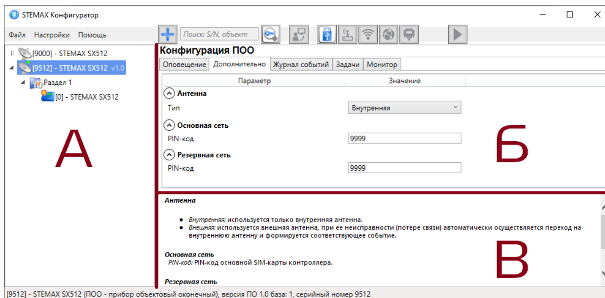
Рисунок 4.6 — Структура основного окна программы (А — дерево устройств, Б — область параметров, В — область подсказок)
