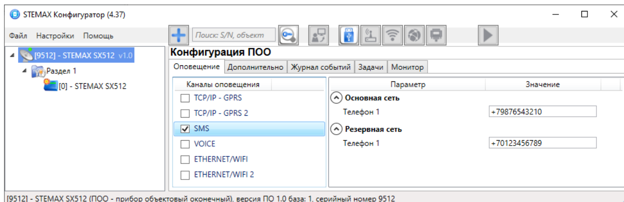
Рисунок 4.19 — Параметры канала SMS
