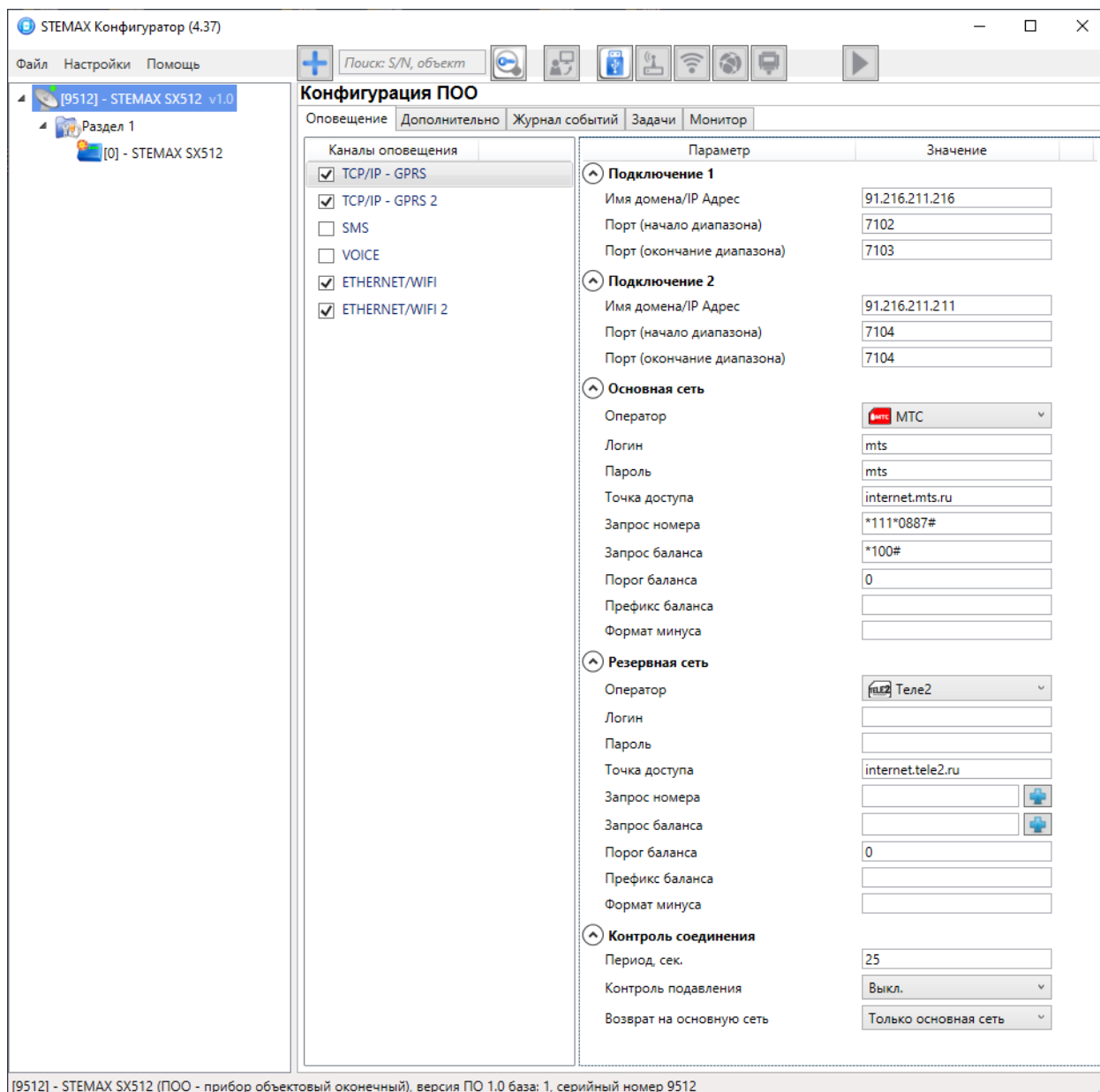
Рисунок 4.17 — Параметры канала TCP/IP – GPRS
