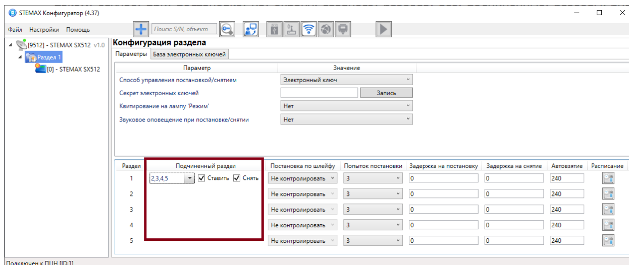
Рисунок 4.32 — Пример 2
