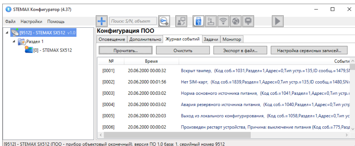
Рисунок 4.24 — Вкладка Журнал событий
